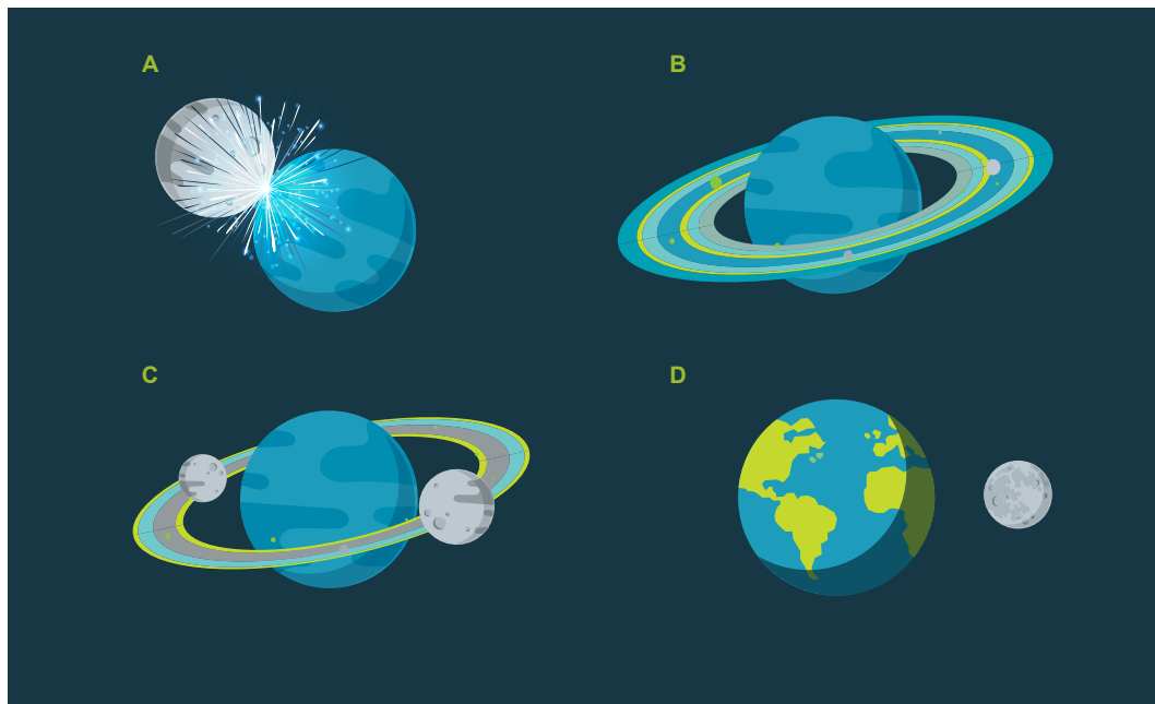
6 Formación de la Luna Fuente: tomada y modificada a partir de Erickson (2003)
