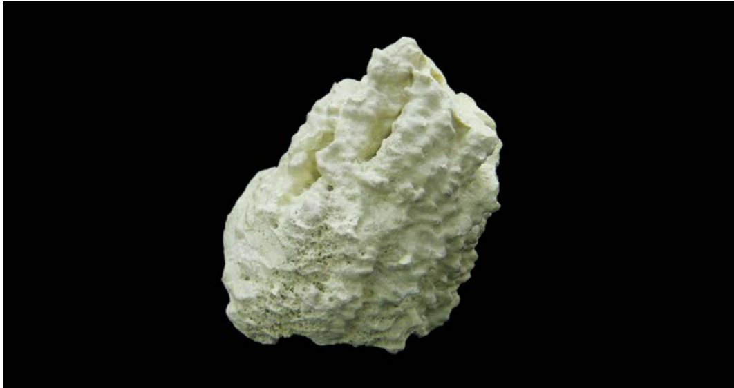
31 Azufre Fuente: Museo SGC
