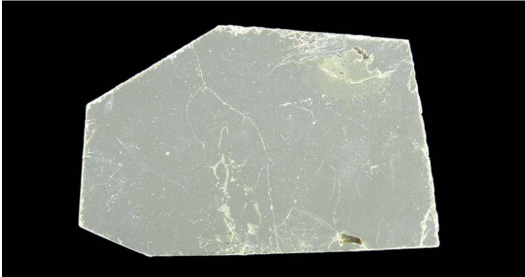
58 Mica, variedad moscovita Fuente: Museo SGC
