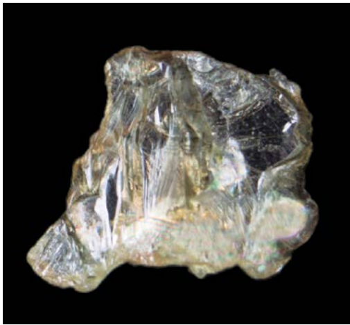
48 Topacio (dureza 8) Fuente: Museo SGC
