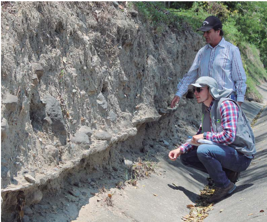
160 Afloramiento del lahar de 1985, con registro de elementos del Holoceno (vestigios de la antigua carretera) en la intersección de la carretera Ibagué-Mariquita, Cambao-Bogotá Fuente: Estefanía Salgado
