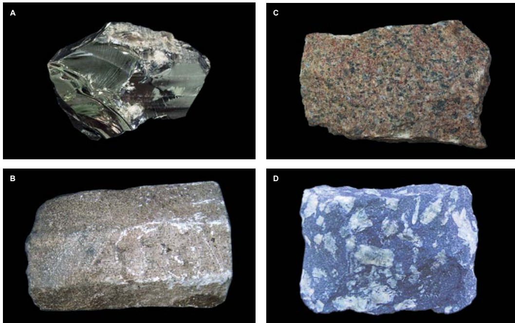
64 Texturas de las rocas ígneas: A. Textura vítrea (obsidiana); B. Textura afanítica; C. Textura fanerítica (granito); D. Textura porfirítica (diabasa porfirítica) Fuente: Museo SGC
