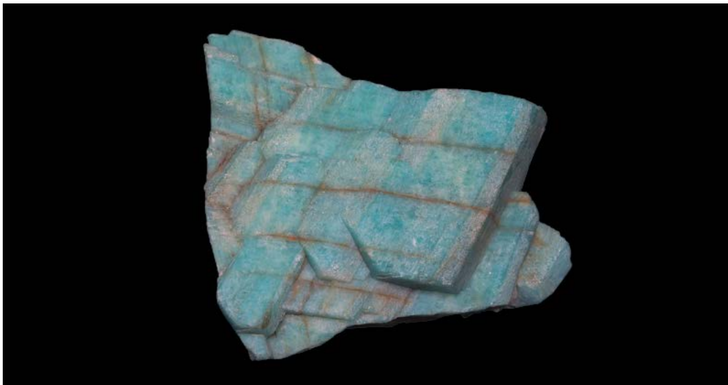
26 Microclina, variedad amazonita Fuente: Museo SGC
