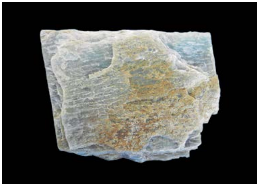
109 Feldespato (microclina) Fuente: Museo SGC
