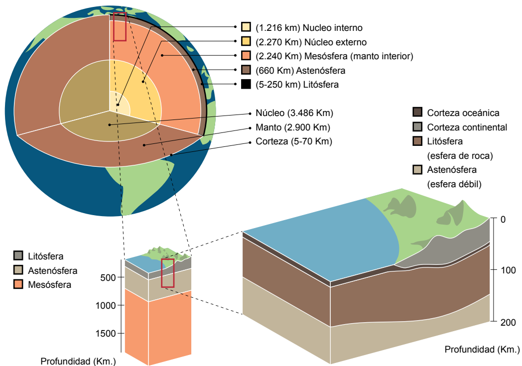
8 Capas de la estructura interna de la Tierra. La parte central ilustra la división según propiedades químicas, y la parte superior derecha, la división según propiedades físicas Fuente: tomada y modificada a partir de Tarbuck y Lutgens (2005)
