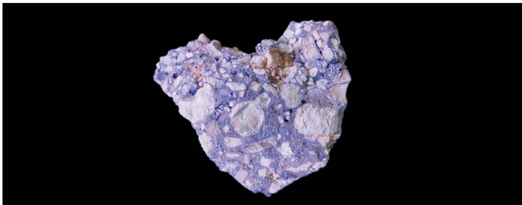
82 Brecha Fuente: Museo SGC
