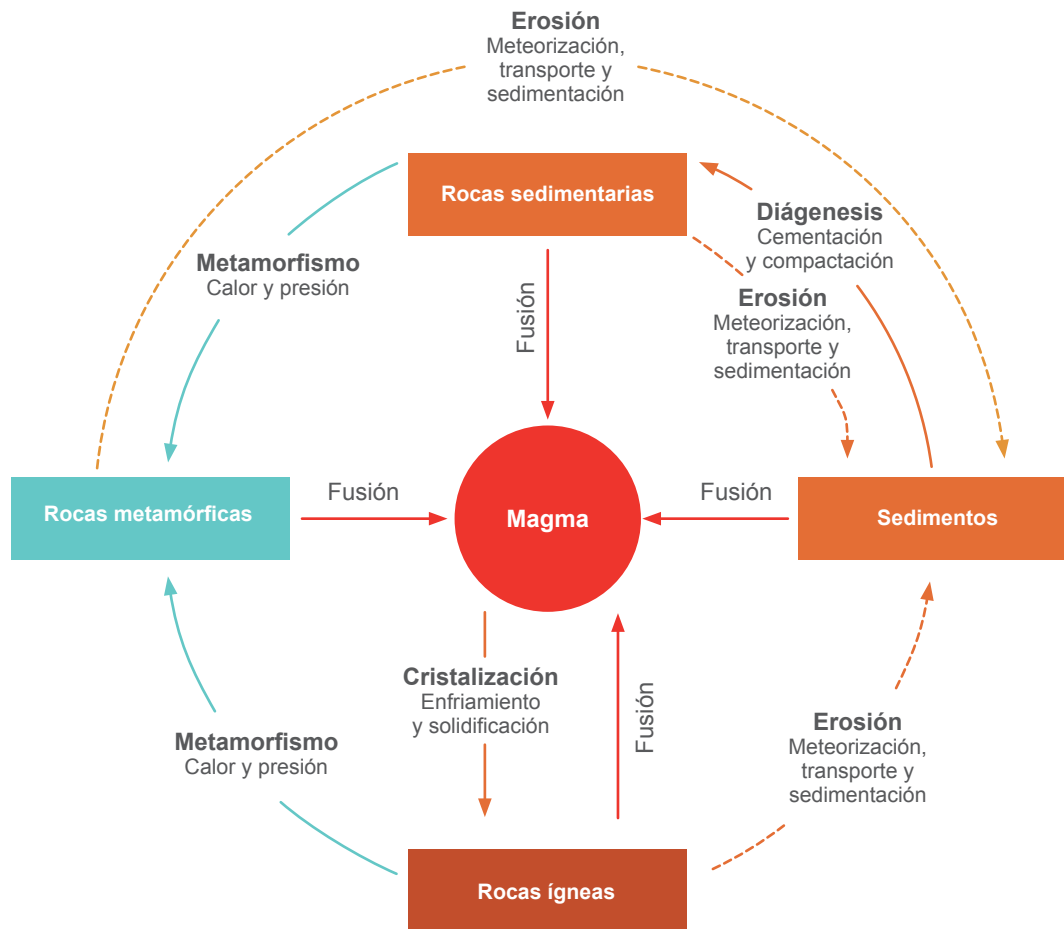
61 Ciclo de las rocas Fuente: tomada y modificada a partir de Agencia Nacional de Hidrocarburos (2009)
