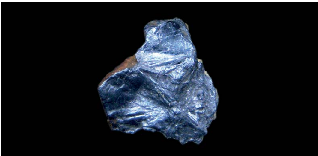
21 Grafito (mineral de carbono) Fuente: Museo SGC
