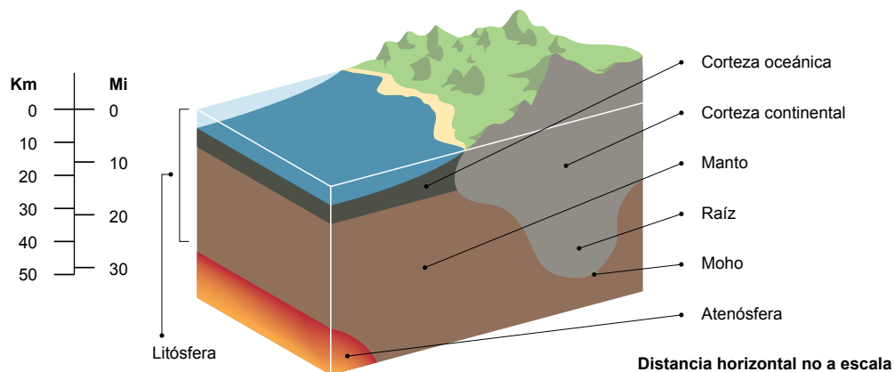
7 Estructura de la parte superior de la Tierra Fuente: tomada y modificada a partir de Stanley (2009)
