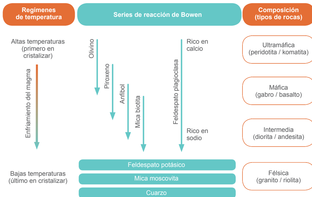
62 Serie de Bowen Fuente: tomada y modificada a partir de Tarbuck y Lutgens (2005)
