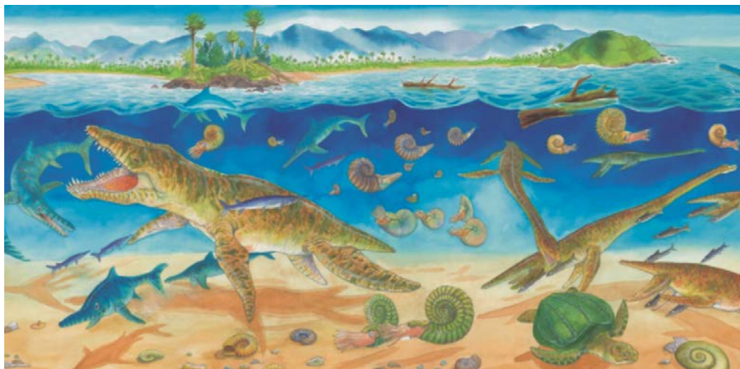
155 Pliosaurio, plesiosaurios, ictiosaurios, tortuga marina y amonitas. Ilustración del mar del cretácico inferior en el área de Villa de Leiva, Boyacá Fuente: Ilustración de Jorge Moreno Bernal para el Museo Geológico SGC. 2007
