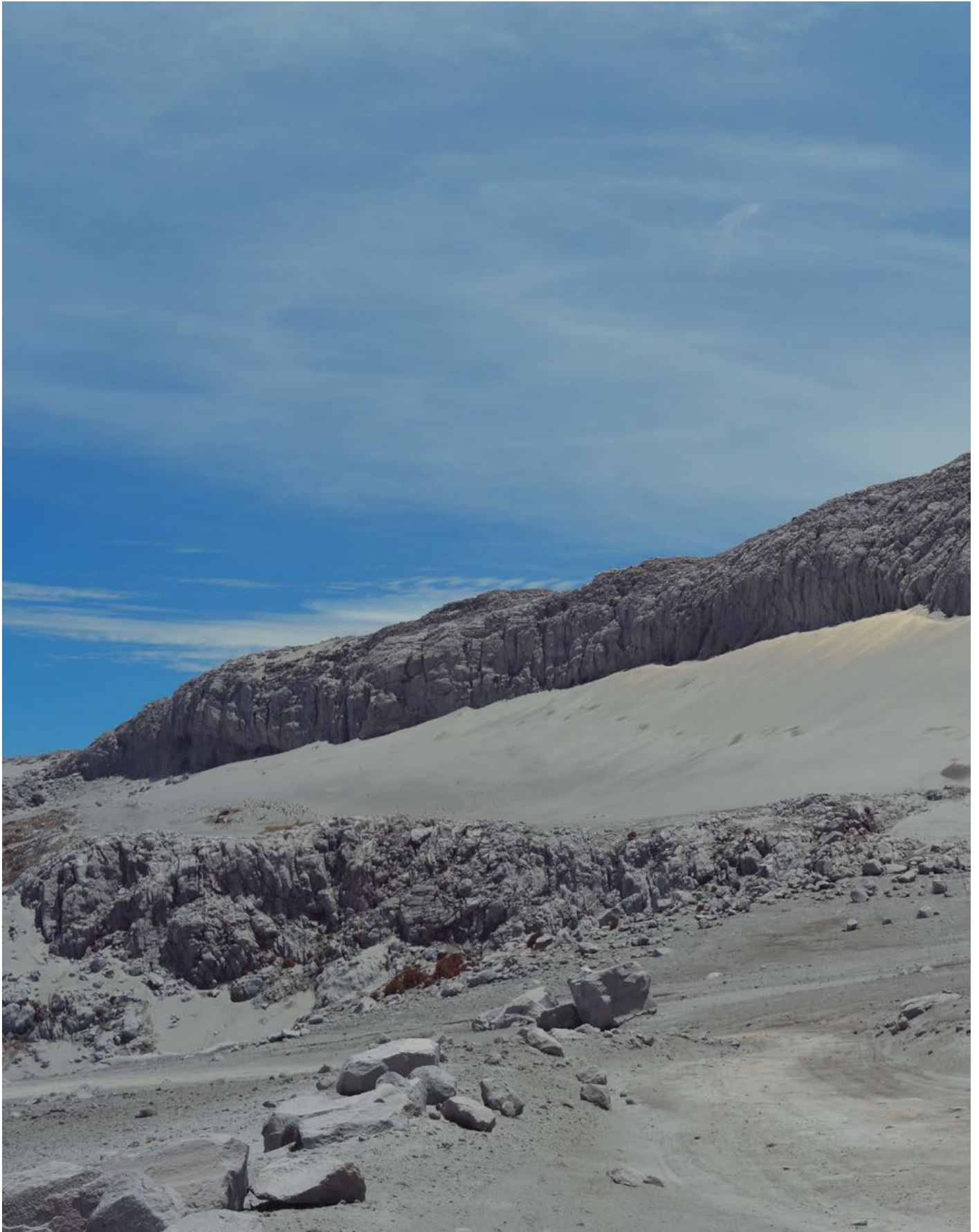
Flujos de lava del Volcán Nevado del Ruiz Fuente: Jair Ramírez Cadena
