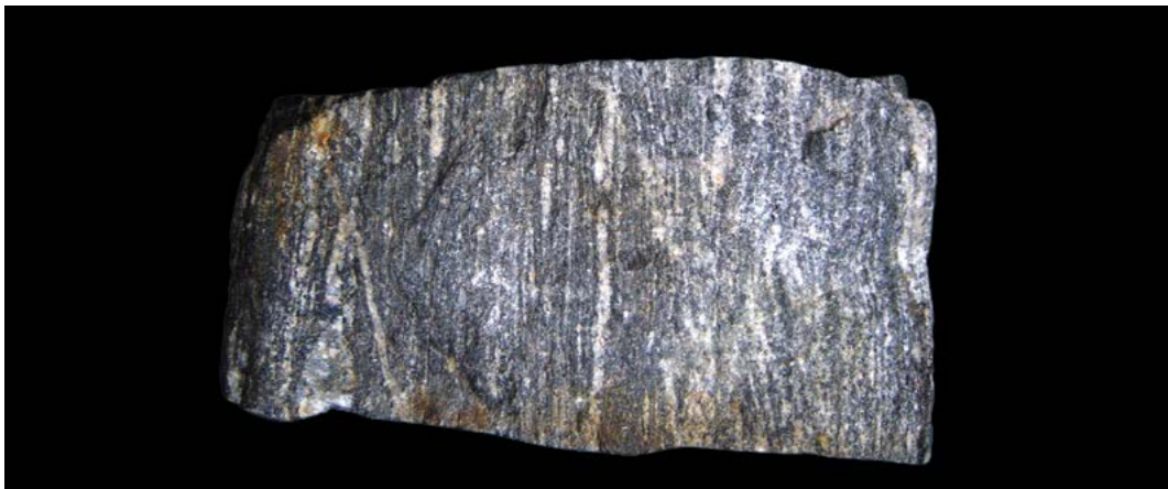
89 Neis Fuente: Museo SGC
