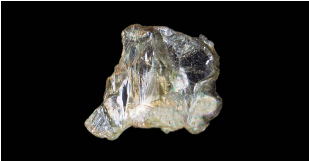
106 Topacio Fuente: Museo SGC
