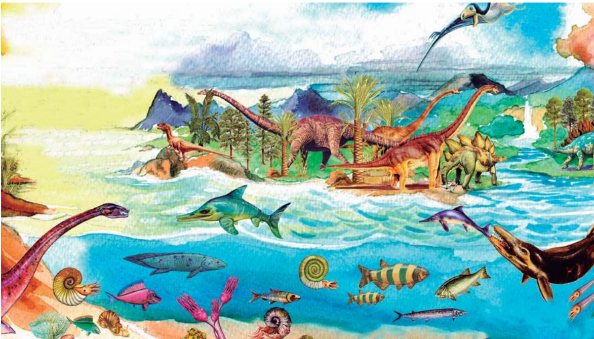
154 Paisaje marino y terrestre del Jurásico Fuente: ilustración de Jhon Fredy Umaña y María Páramo para el Museo Geológico SGC. 2001
