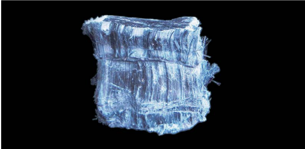
33 Crocidolita (asbesto azul, silicato) Fuente: Museo SGC
