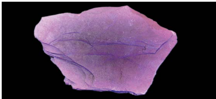
96 Pizarra Fuente: Museo SGC
