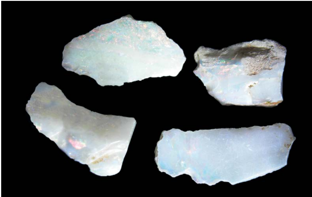
40 Ópalo (mineraloide de sílice). Al difractarse, la luz produce en la superficie del mineral una serie de colores parecidos al arco iris Fuente: Museo SGC
